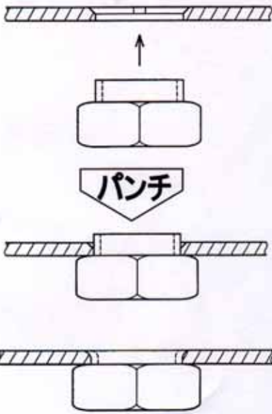
【かしめ方法】
